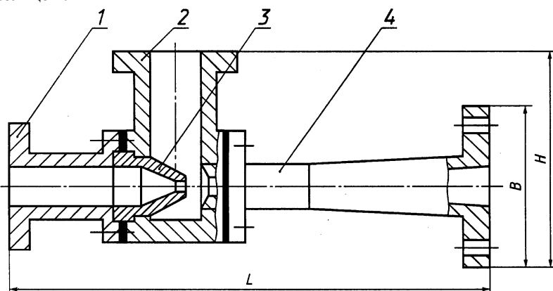
1 — входной патрубок, 2 — всасывающая камера, 3 — сопло, 4 — выходной патрубок
