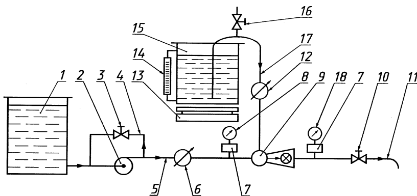
1 - емкость для воды; 2 - насос; 3 - вентиль; 4 - обводное кольцо на насосе; 5 - напорный трубопровод; 6, 12 - водомер; 7 - демпфирующее устройство под манометром; 8, 18 - манометры; 9 - дозатор; 10 - вентиль; 11 - сливной патрубок; 13 - весы; 14 - уровнемер; 15 - бак для пенообразователя (добавки); 16 - вентиль; 17 - всасывающий трубопровод для пенообразователя
